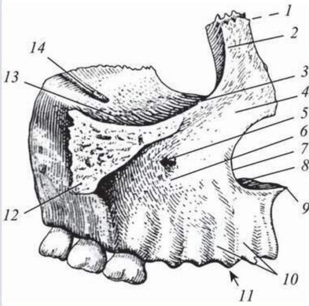
Рис. 2. Верхнечелюстная кость, правая (вид снаружи):
