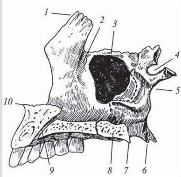
Рис. 3. Верхнечелюстная кость, правая (вид изнутри):
